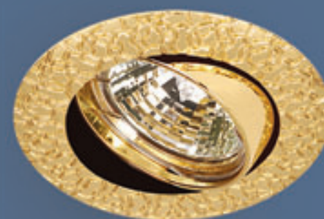
625 SG (сатинованное золото) MR16 G5.3 max 50 Вт Ø 86 мм h 75 мм
