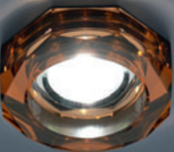
9120 BROWN (коричневый) MR16 G5.3 max 50 Вт Ø 90 мм 65 мм
