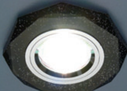
8020/2 BK/SL (черный / хром) MR16 G5.3 max 50 Вт Ø 90 мм 65 мм
