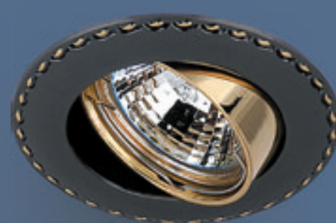
635 GMG (черный / золото) MR16 G5.3 max 50 Вт Ø 86 мм h 75 мм
