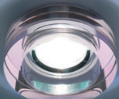
9160 PK (розовый) MR16 G5.3 max 50 Вт Ø 90 мм 65 мм
