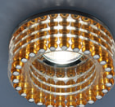
722 BR (янтарь) MR16 G5.3 max 50 Вт \varnothing 100 мм \bar{h} 55 мм
