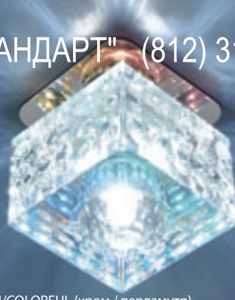
8247 CH/COLORFUL (хром / перламутр) G9 max 50 Вт 68 × 68 мм \bar{h} 55 мм
