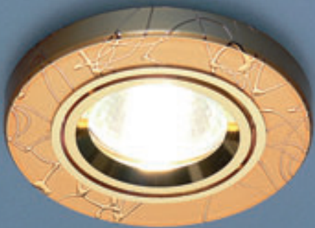
2050/2 GD (золото) MR16 G5.3 max 35 Вт Ø 90 мм 65 мм
