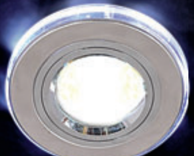
2060/2 SL/LED/WH (хром / белый) MR16 G5.3 max 35 Вт Ø 90 мм Ъ 65 мм
