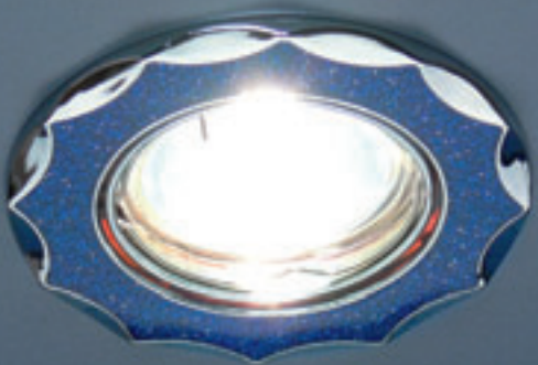
612A SH BL/2 (синий блеск / хром) MR16 G5.3 max 50 Вт Ø 85 мм 75 мм
