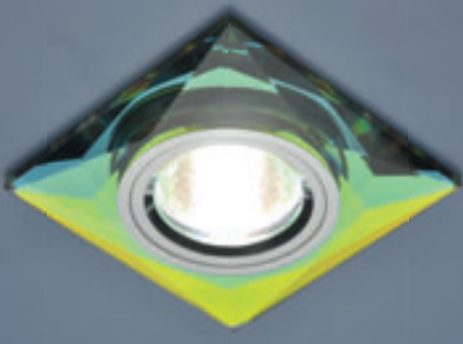
8470 MULTI/CH (зеркальный / мультицвет) MR16 G5.3 max 50 Вт 90 x 90 мм 65 мм
