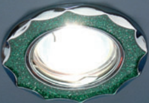
612A SH GR (зеленый блеск / хром) MR16 G5.3 max 50 Вт Ø 85 мм 75 мм
