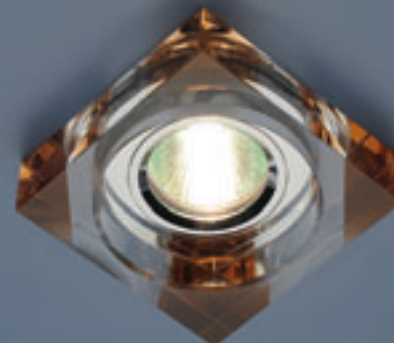
700S BROWN BICOLOR (коричневый) MR16 G5.3 max 50 Вт 90 x 90 мм 60 мм
