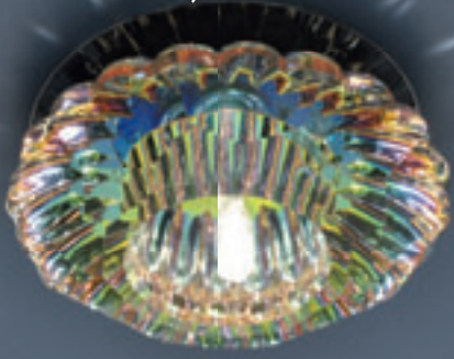
8180 MULTI (мульти) G4 max 40 Вт Ø 107 мм H 50 мм
