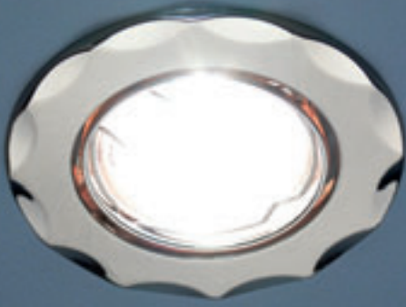
734 SN/N (сатиновый никель / никель) MR16 G5.3 max 50 Вт Ø 88 мм 75 мм
