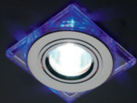
2080 CH/BL (хром / синий) MR16 G5.3 max 35 Вт 90 × 90 мм H 65 мм
