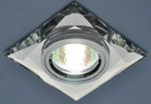
8470 CLEAR/CH (зеркальный / серебро) MR16 G5.3 max 50 Вт 90 x 90 мм 65 мм
