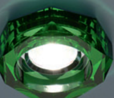
9120 GR (зеленый) MR16 G5.3 max 50 Вт Ø 90 мм 65 мм
