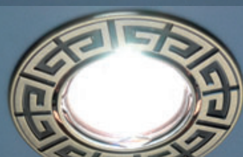
120090 SB (бронза) MR16 G5.3 max 50 Вт Ø 92 мм 75 мм
