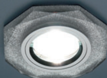
8020/2 BR/SL (серебряный блеск) MR16 G5.3 max 50 Вт Ø 90 мм 65 мм
