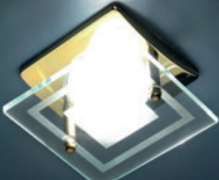
R50D GD (золото) E14 R50 max 50 Вт 95 × 95 мм H 125 мм H 70 мм
