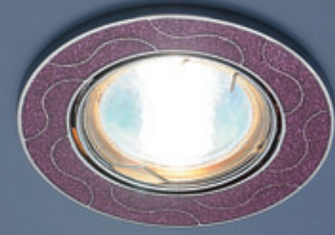
616 SP/CH (блеск сиреневый / хром) MR16 G5.3 max 50 Вт Ø 86 мм 75 мм
