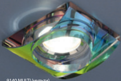
9140 MULTI (мульти) MR16 G5.3 max 50 Вт 100 x 80 x 40 мм 63 мм
